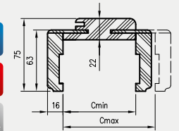
Przekrój OR/ORC z ką. K63
