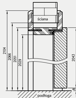
Przekrój pionowy drzwi przylgowych OR
