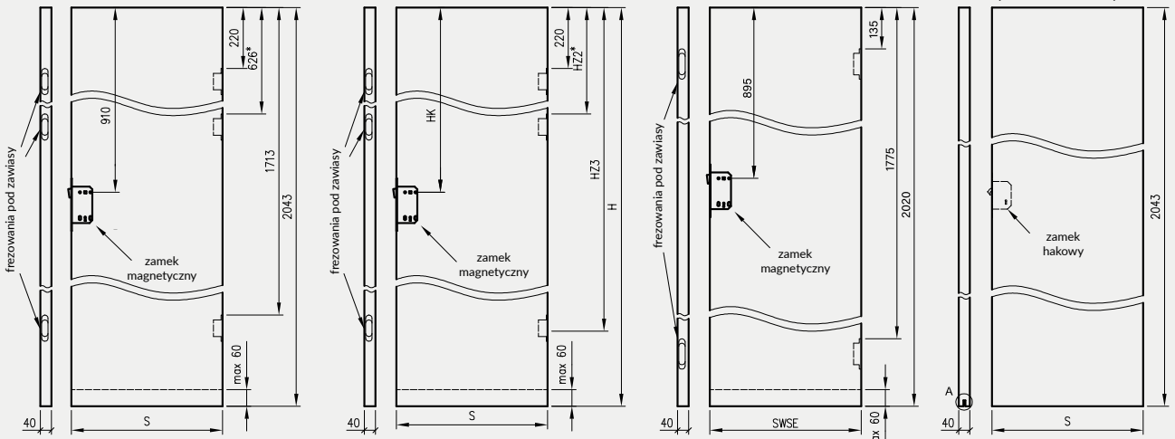
Skrzydła przesuwne do: - kaset ościeżnicowych PA - systemów SPAZIO CD - systemów naściennych
