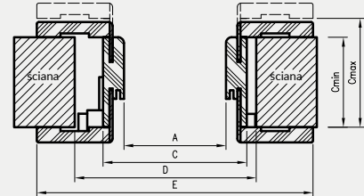
Przekrój poziomy ORB
