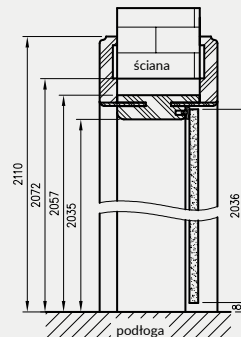
Przekrój pionowy drzwi szklanych ORC
